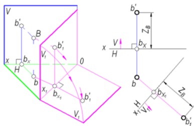
Замена фронтальной плоскости V новой плоскостью проекций V_1
