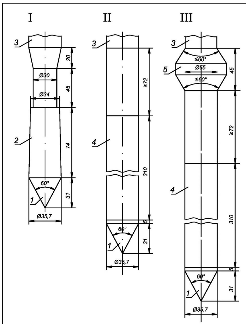
Рис.33. Зонды для статического зондирования I, II и III типа 1 – конус; 2 – кожух; 3 – штанга; 4 – муфта трения; 5 – уширитель
