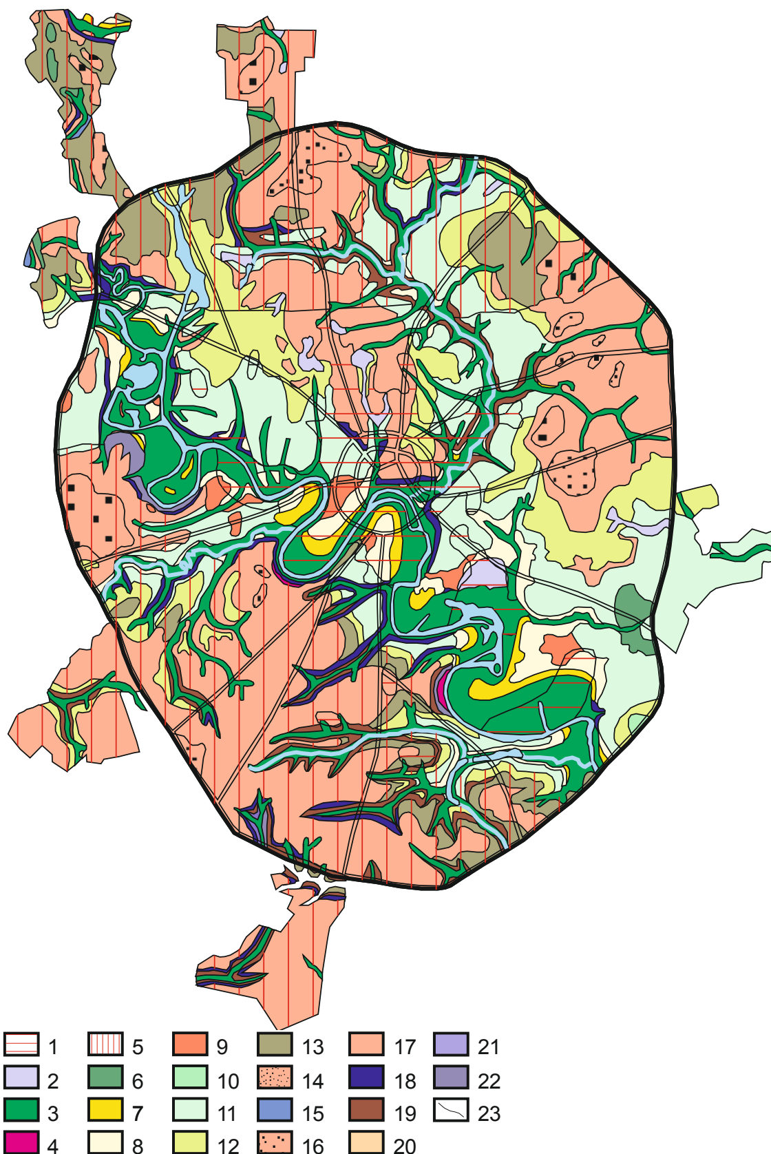
Рис. 8. Геологическая карта четвертичных отложений и образований (составила О.А. Лавровиц по материалам Е.А. Шулешкиной и И.В. Фурсиковой, 1997).
