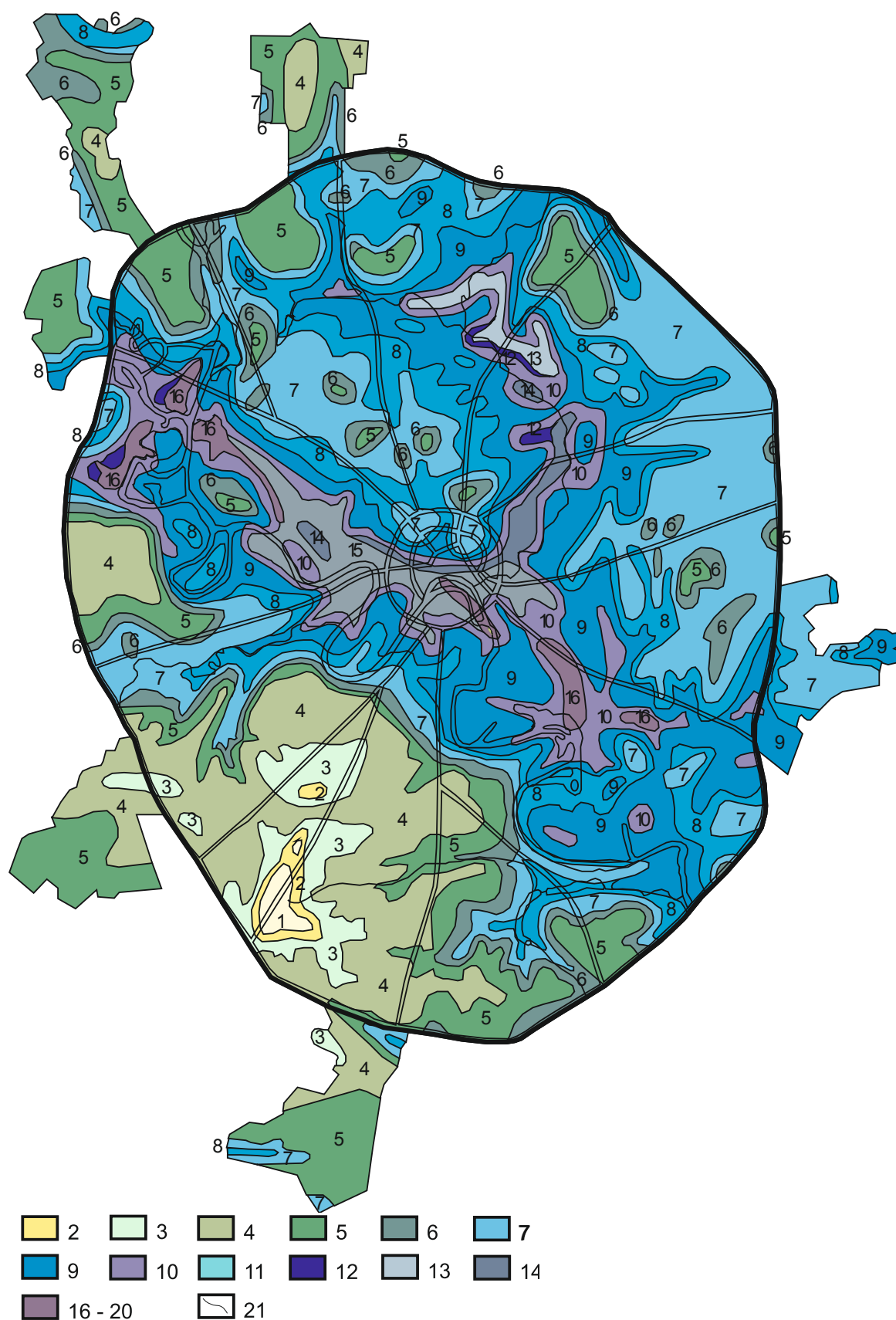
Рис. 7. Геологическая карта дочетвертичных образований (составила Е.А. Гаврюшова по материалам Е.С. Артемьевой, 1996).
