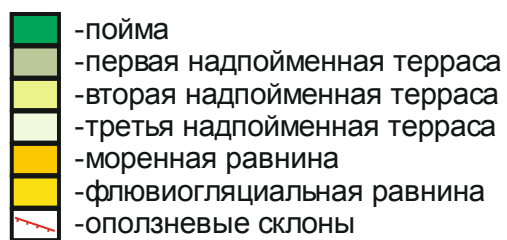
Рис. 4. Геоморфологическая схема г. Москвы (В.И. Осипов, О.П. Медведев и др., 1997)
