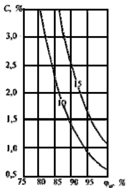
Рисунок Ф.2 - Изолинии сорбционного влагосодержания керамзитобетона плотностью \rho_p = 1200 \text{ кг/м}^3 , содержащего хлорид калия, при изменении относительной влажности воздуха \varphi_{\text{в}} , %, и массового солесодержания C , %
