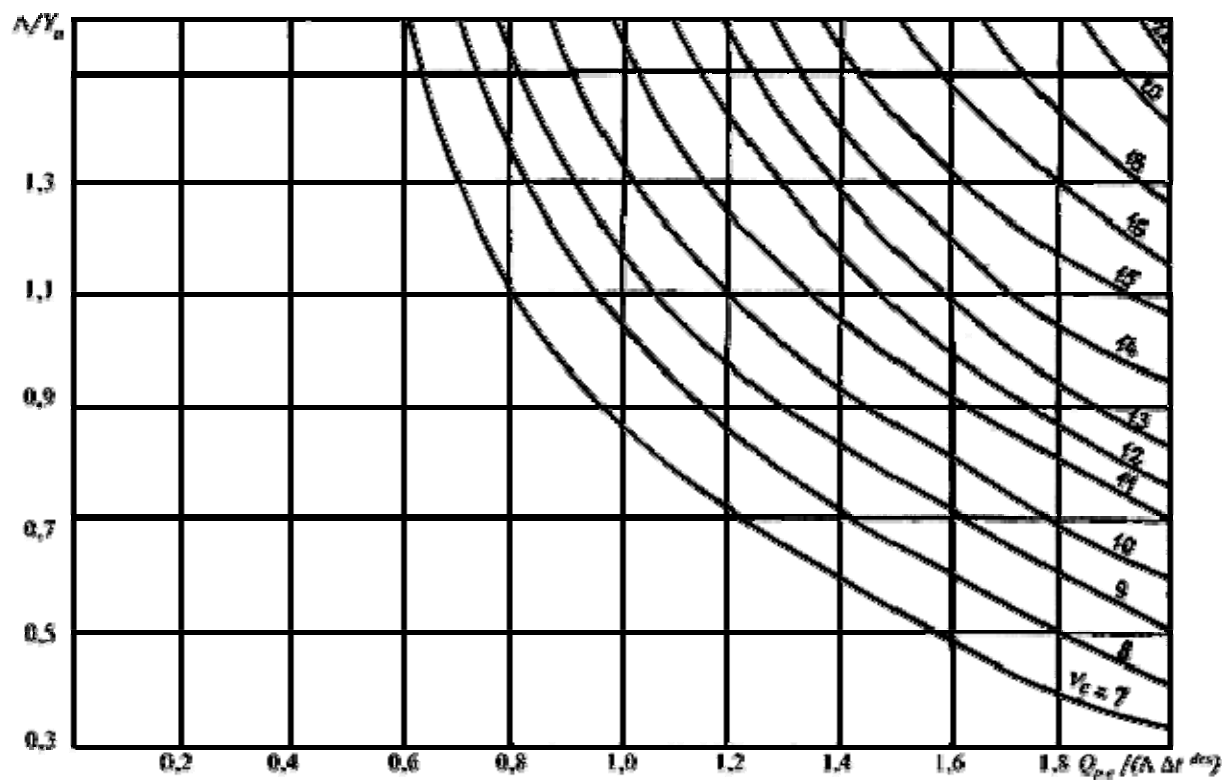
Рисунок 3 - График для подбора теплоаккумулирующих приборов (продолжительность m зарядки 6 ч + 2 ч дневной подзарядки)
