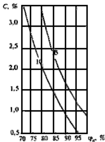
Рисунок Ф.4 - Изолинии сорбционного влагосодержания керамзитобетона \rho_b=1200 \text{ кг/м}^3 , содержащего NaCl - 60%, KCl - 30%, \text{MgCl}_2 - 10%, при изменении относительной влажности воздуха \varphi_{\text{в}} , %, и массового солесодержания C , %, в стенах флотофабрик
