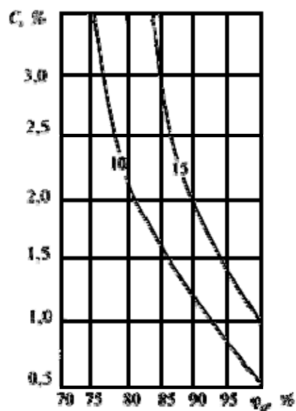
Рисунок Ф.5 - Изолинии сорбционного влагосодержания керамзитобетона \rho_s = 1200 \text{ кг/м}^3 , содержащего NaCl - 50%, KCl - 30%, \text{MgCl}_2 - 20%, при изменении относительной влажности воздуха \varphi , %, и массового солесодержания C , %, в стенах цехов дробления руды
