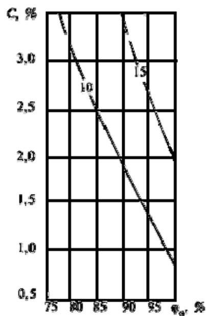
Рисунок Ф.3 - Изолинии сорбционного влагосодержания керамзитобетона \rho_b=1200 \text{ кг/м}^3 , содержащего хлорид магния, при изменении относительной влажности воздуха \varphi_{\text{в}} , %, и массового солесодержания C , %
