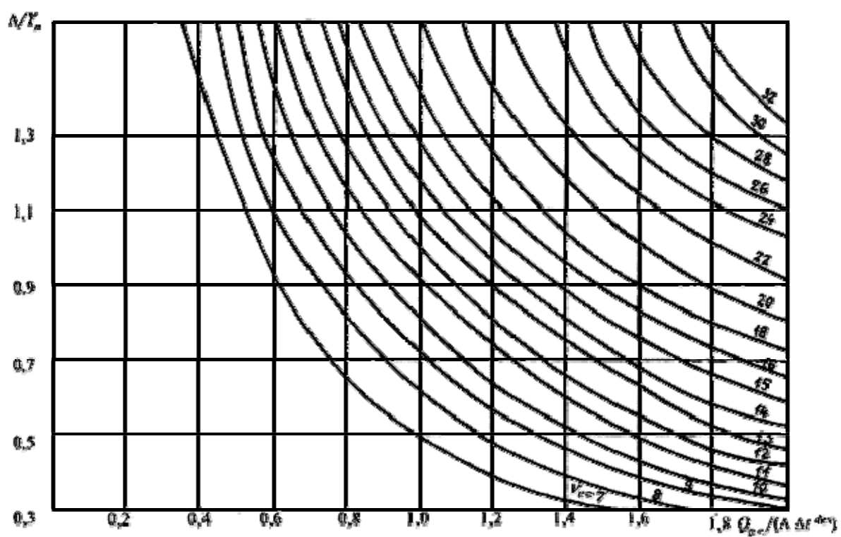
Рисунок 1 - График для подбора теплоаккумулирующих приборов (продолжительность m зарядки 8 ч)
