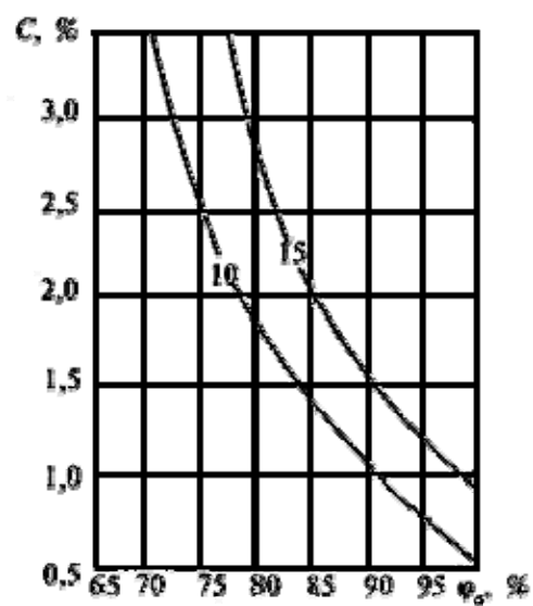
Рисунок Ф.1 - Изолинии сорбционного влагосодержания керамзитобетона плотностью \rho_p = 1200 \text{ кг/м}^3 , содержащего хлорид натрия, при изменении относительной влажности воздуха \varphi_{\text{в}} , %, и массового солесодержания C , %
