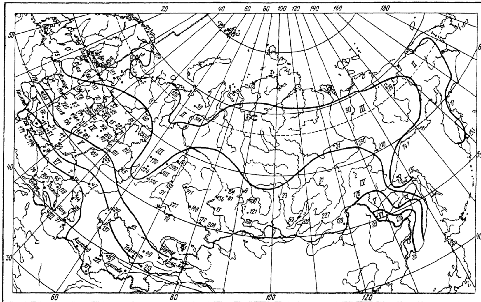
Карта-схема 1-го районирования территории СССР по величине удельной энтальпии I , кДж/кг, наружного воздуха в теплый период года (параметры A ) для районов
