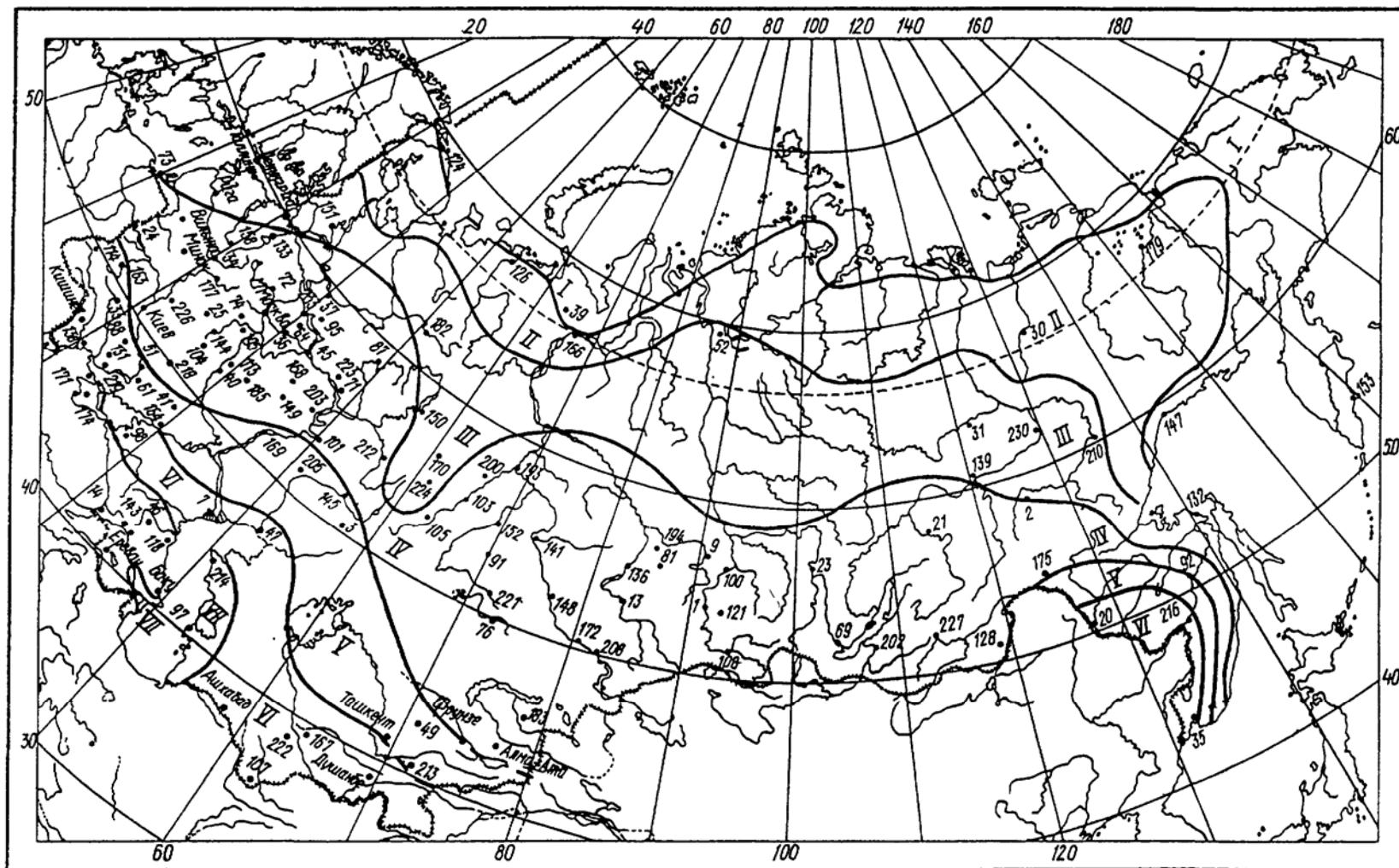
Карта-схема 2-го районирования территории СССР по величине удельной энтальпии I , кДж/кг, наружного воздуха в теплый период года (параметры Б) для районов
