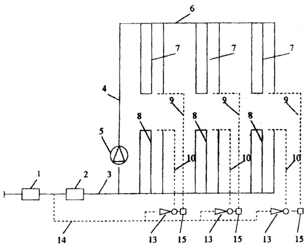
Рис. 4.1. Принципиальная схема двухзонной системы горячего водоснабжения с элеваторным побуждением циркуляции в нижней зоне Схемы: "а" - с общим элеватором; "б" - с элеватором в каждой секции.
