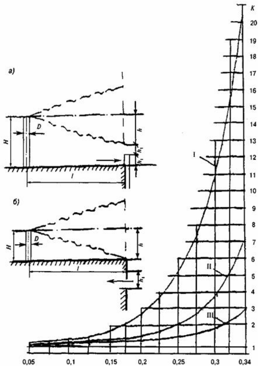
а - расположение источника над зоной всасывания наружного воздуха приемным устройством (высота трубы источника H = 2h_l + h ); б- то же, над кровлей здания (высота трубы
