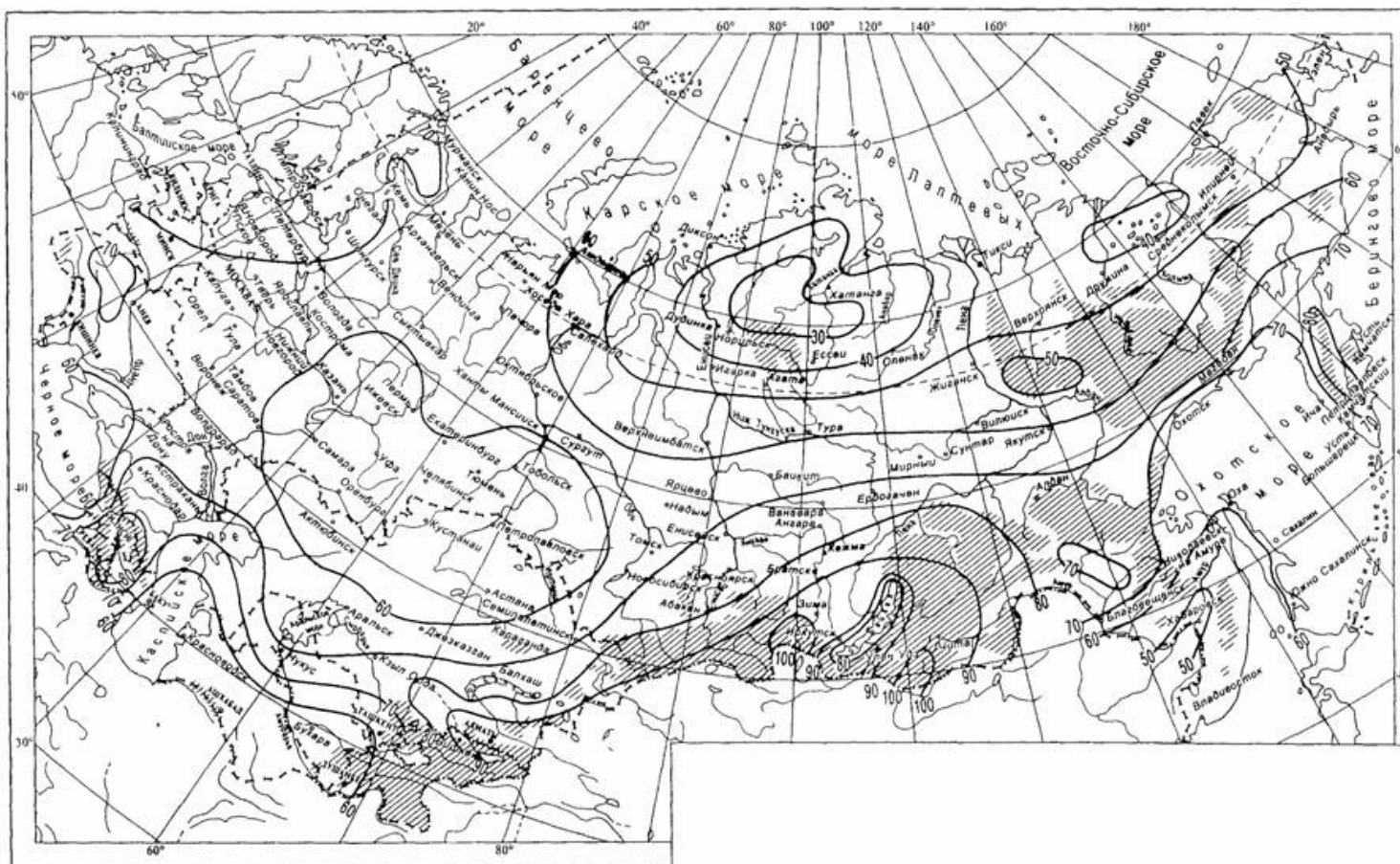
Рисунок 4 - Схематическая карта распределения среднего за год числа дней с переходом температуры воздуха через 0 °C (рекомендуемая)
