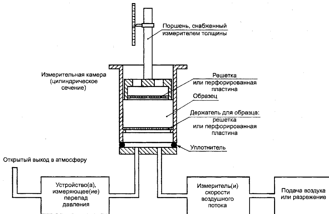
Рисунок Б.3 — Схема установки с цилиндрической измерительной камерой для определения сопротивления продуванию методом А
