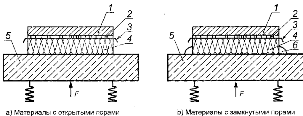
Рисунок Г.1 — Схема возбуждения нагружающей пластины. Измерение вибрации нагружающей пластины
