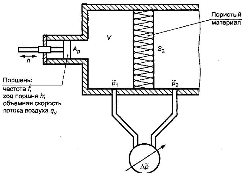
Рисунок Б.2 — Схема определения сопротивления продуванию переменным потоком воздуха (метод В). Основной принцип
