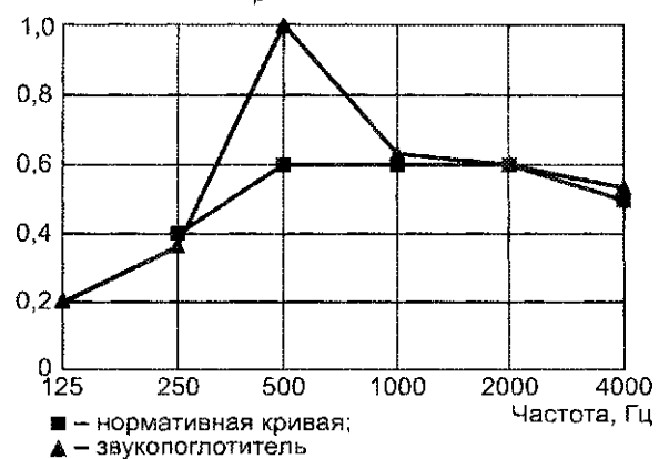
Рисунок В.4 — Пример определения индекса звукопоглощения с применением индикатора формы \alpha_w [\alpha_w = 0,60 (M)]
