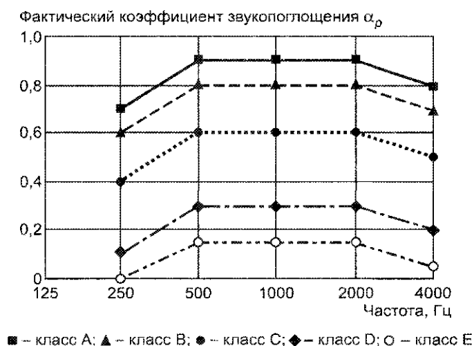
Рисунок 1 — Нормативные кривые, ограничивающие классы звукопоглощения
