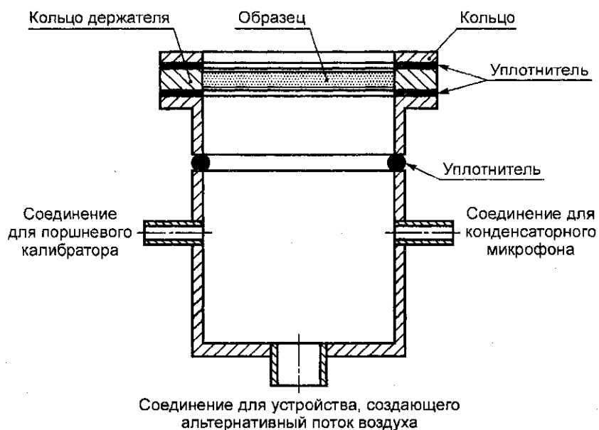
Рисунок Б.5 — Схема измерительной камеры с держателем для цилиндрического образца (метод В)
