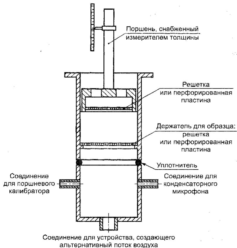
Рисунок Б.4 — Схема измерительной камеры, снабженная держателем для образца, изготовленного из волокнистого сыпучего материала или материала плотной структуры (метод В)
