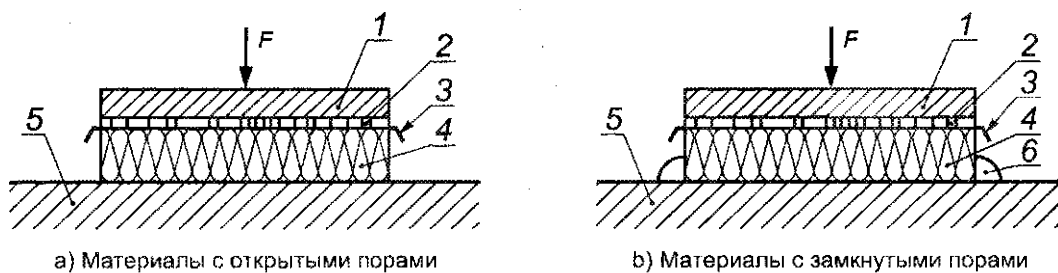
Рисунок Г.1 — Схема возбуждения нагружающей пластины. Измерение вибрации нагружающей пластины
