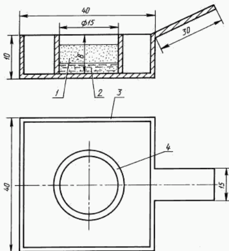
1 — песок; 2 — жидкость; 3 — лодочка; 4 — цилиндрическая емкость
