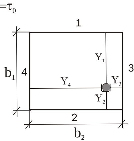
Рис. 2. Расчетная схема прогрева для арматуры при четырехстороннем огневом воздействии.
