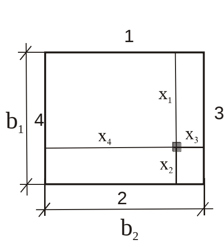
Рис. 1. Расчетная схема прогрева для бетона при четырехстороннем огневом воздействии.
