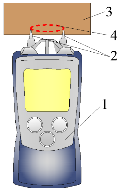
Рис. 1.2. Измерение влажности материала с помощью игольчатого влагомера:
