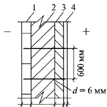
Рис.1. Схема ограждающей конструкции
