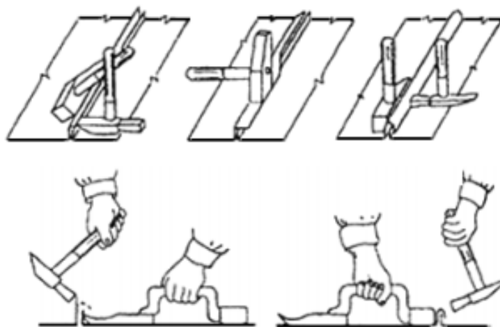
Рис. 1. соединение кровельных картин с помощью молотков и молотка и бруса-отворотки
