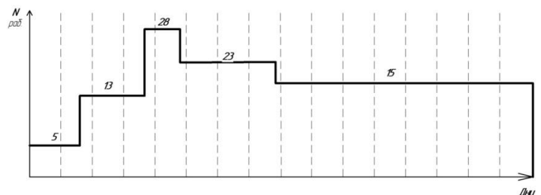
Рис. 1. Календарный график, график движения рабочей силы, коэффициент неравномерности
