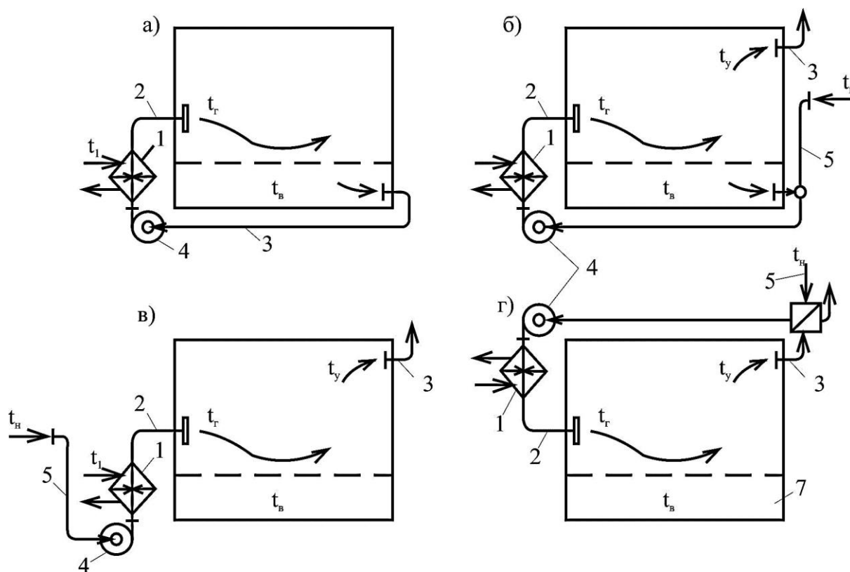
Рисунок 6.5. Принципиальные схемы центральной системы воздушного отопления:
