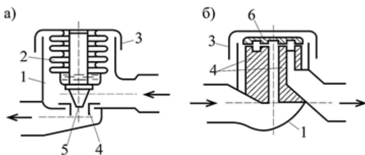
Рисунок 6.3. Конструкция конденсатоотводчиков:
