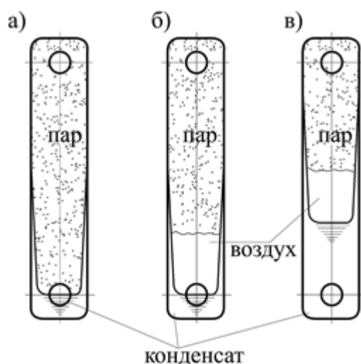
Рисунок 6.1. Распределение пара, конденсата и воздуха в отопительном приборе:
