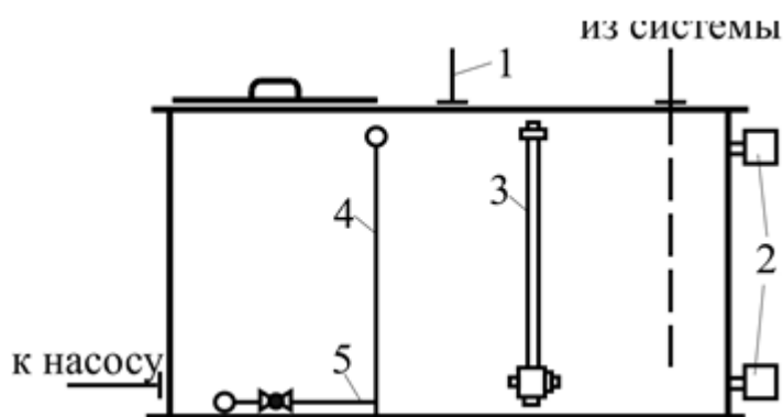
Рисунок 6.4. Конденсатный бак:
