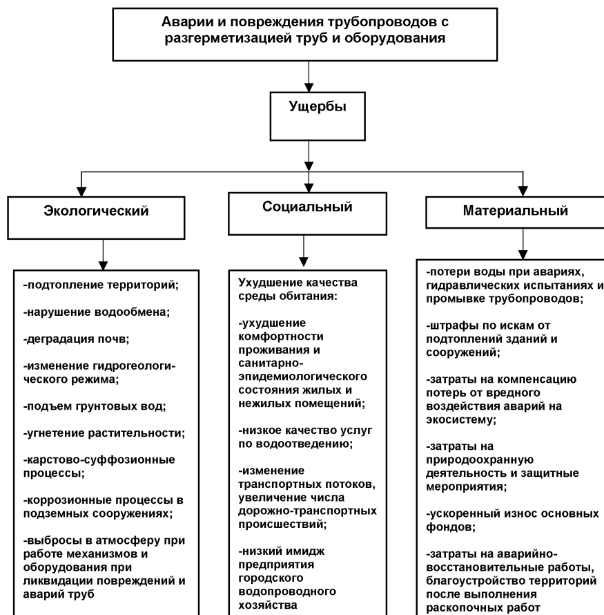
Рис. 1.1.9. Структура ущерба и издержек от повреждений и аварий на трубопроводах
