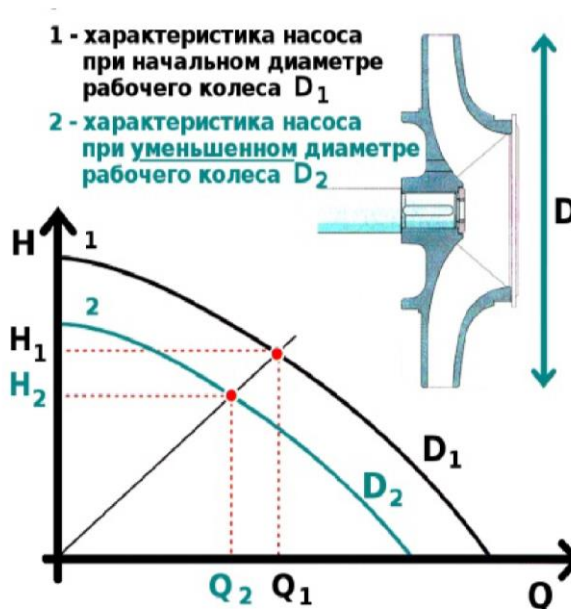
Рис. 1.4.11. Изменение характеристик насоса при коррекции рабочего колеса
