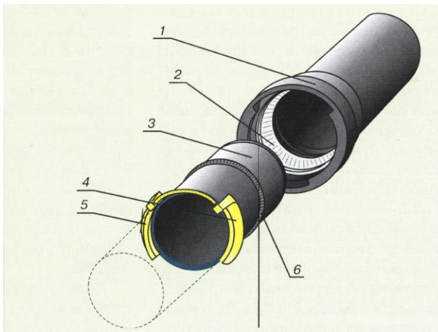
Рис. 1.1.2. Элементы замкового соединения ВРС. 1-раструбная часть трубы, 2-уплотнительная манжета; 3- гладкий конец трубы; 4- стопор правый; 5- стопор левый; 6- наварной валик
