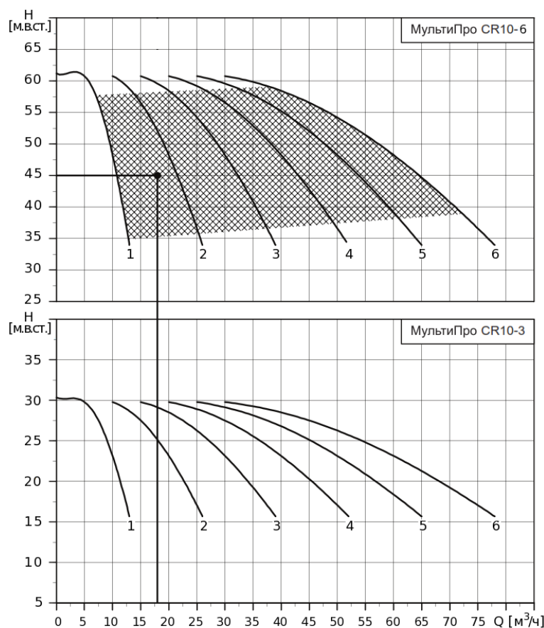
Рис. 1.4.3. Подбор МАНС на рабочую точку характеристики H-Q
