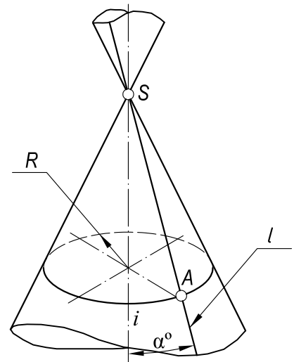
КОНИЧЕСКАЯ ПОВЕРХНОСТЬ
