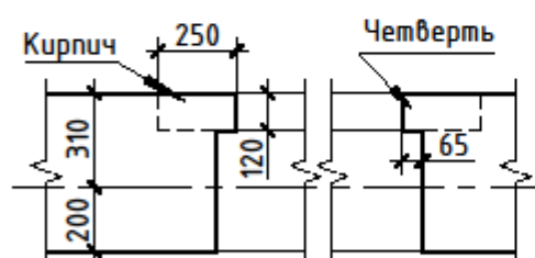
Толщина стен
