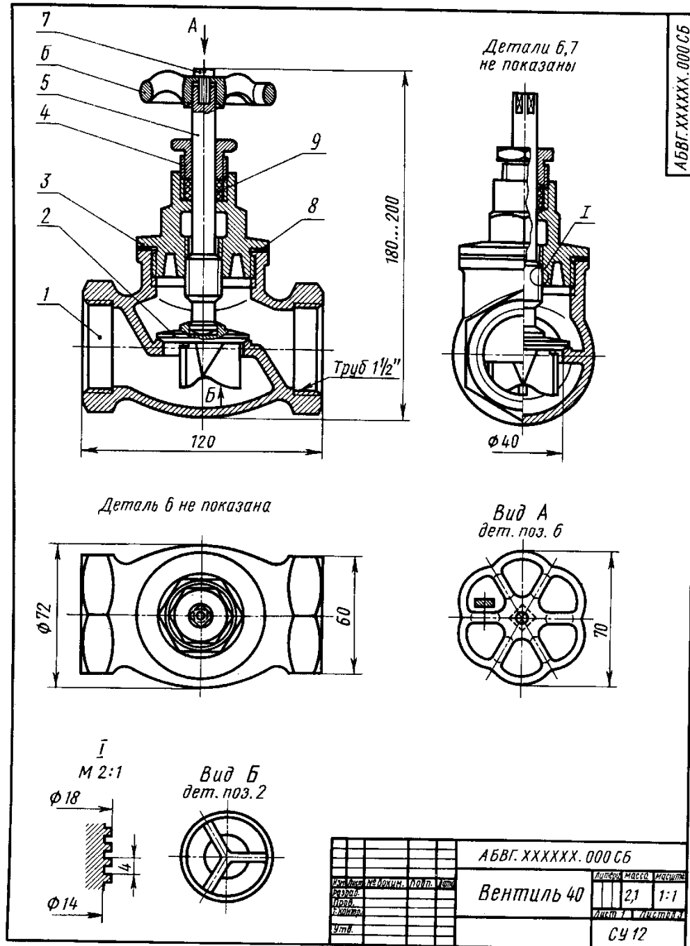
Рис.1 Сборочный чертеж
