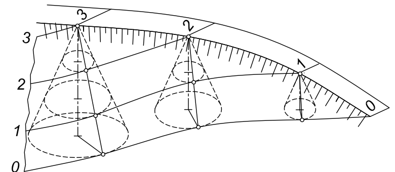
Поверхность одинакового ската
